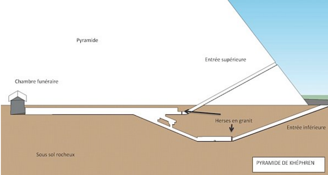
Vue en coupe de la pyramide.
