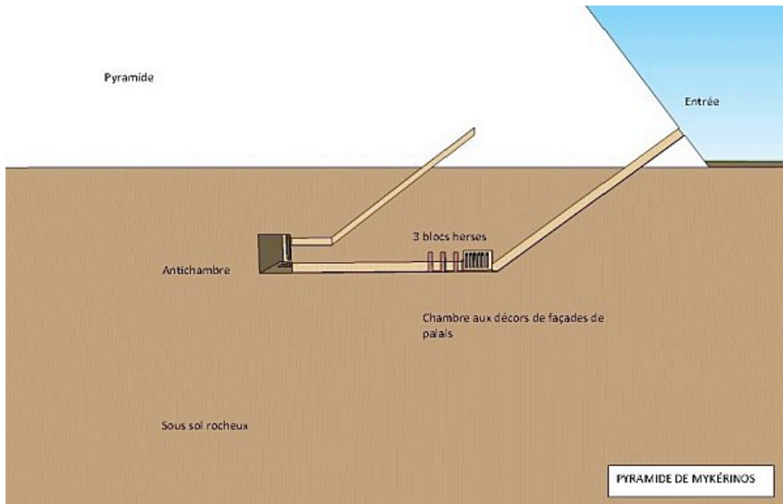
Vue en coupe de la pyramide.
