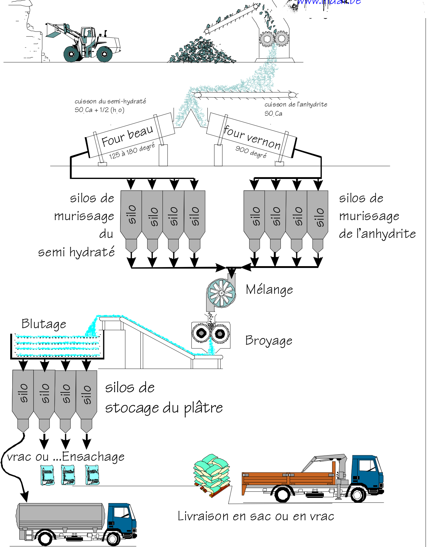
Schéma de fabrication du plâtre
