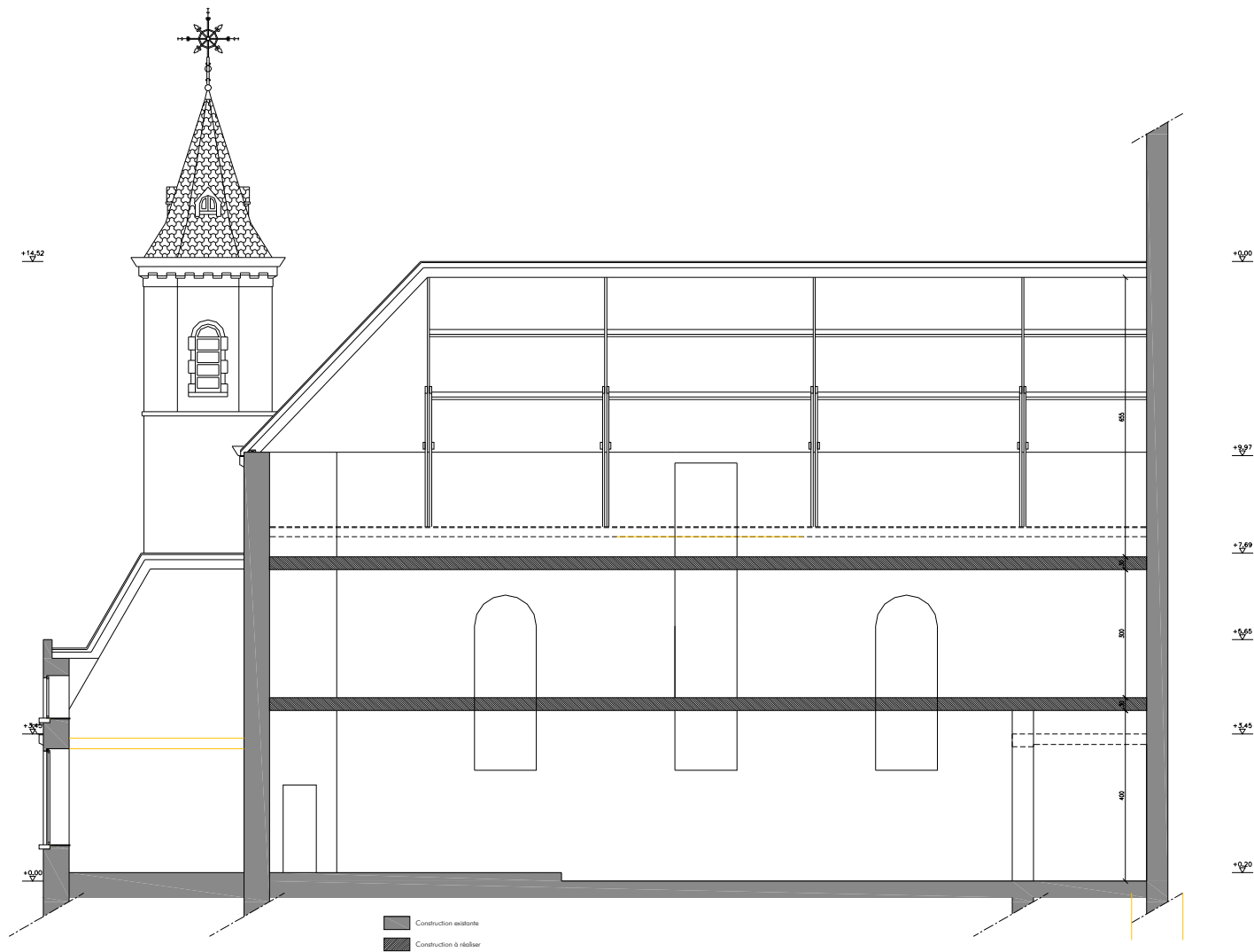
Coupe CC
