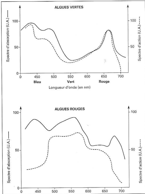
Document 1 Spectres d'absorption et spectres d'action des algues vertes et des algues rouges
