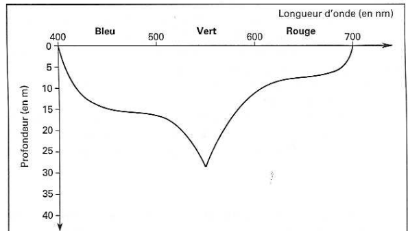
Document 3 Profondeur de disparition des différentes radiations lumineuses dans l'eau
