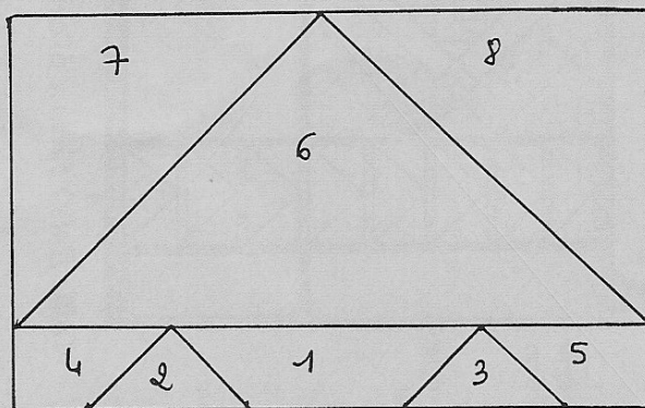
Gabarits taille réelle pour la confection des sangles (coutures non comprises)
