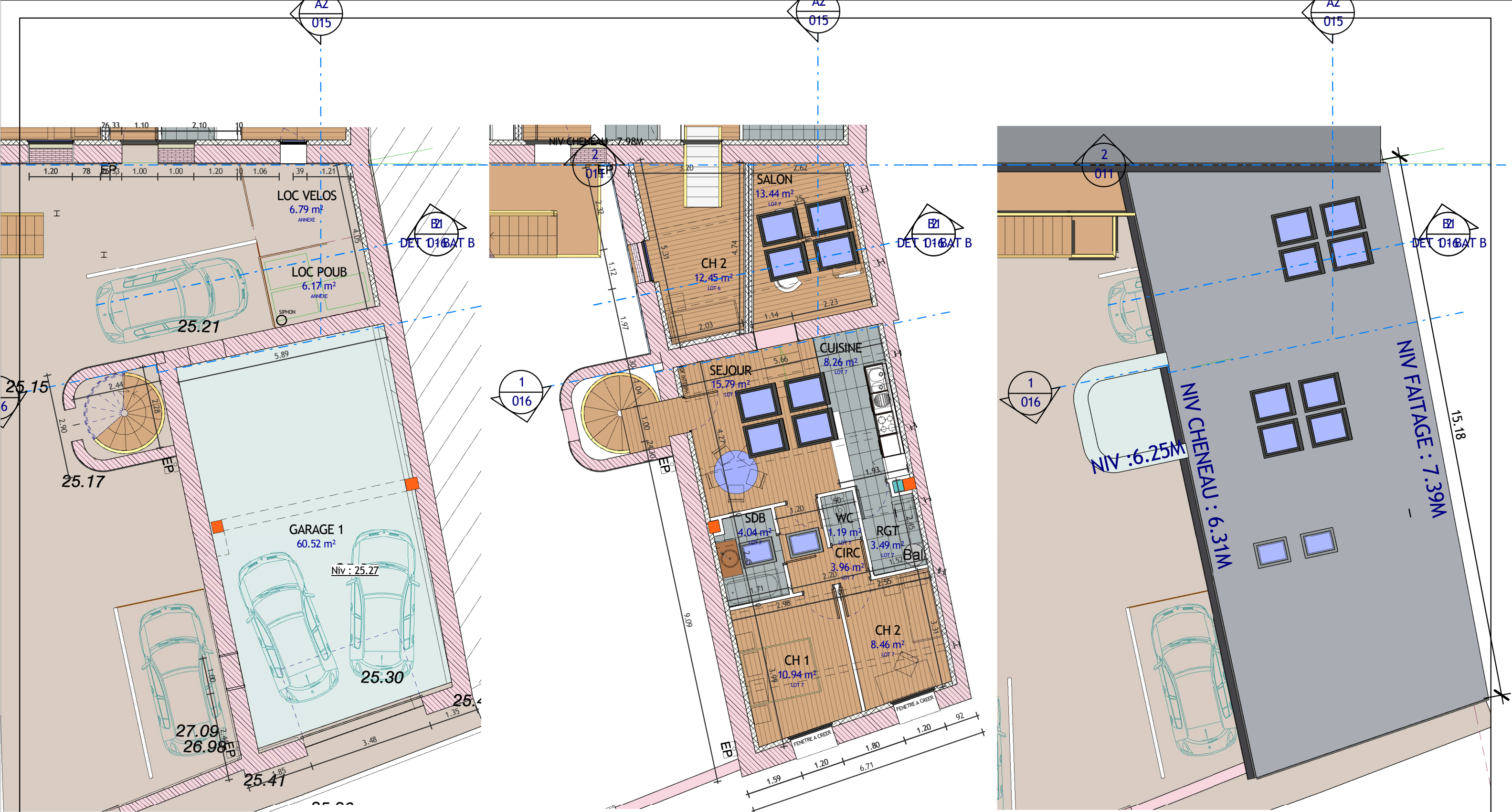
1 Niveau 00 BAT B Ech : 1 : 100
