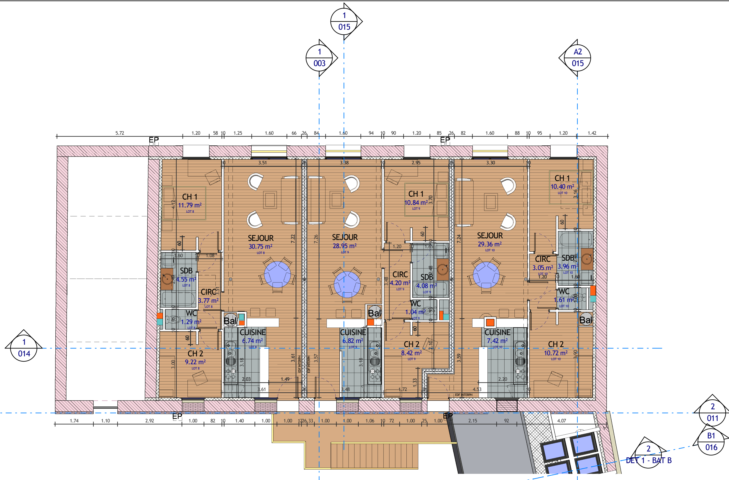
1 02 Niveau 02 BAT A Ech : 1 : 100
