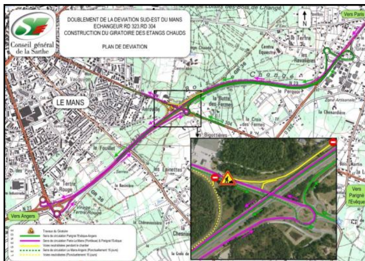
Aménagement du giratoire des Étangs Chauds
