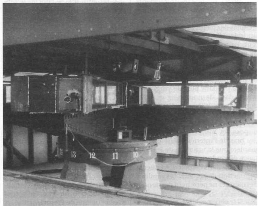
L'interféromètre que Miller utilisa au Mont-Wilson entre 1924 et 1926.
