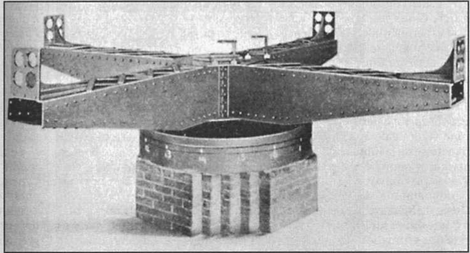
Figure 4 - L'interféromètre de Morley et Miller (1903)
