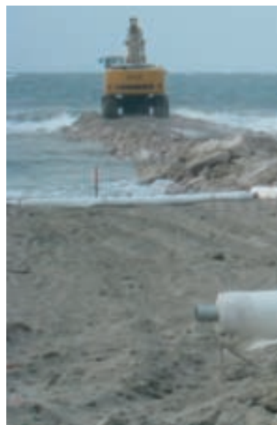
Un ouvrage de protection de 180 mètres
