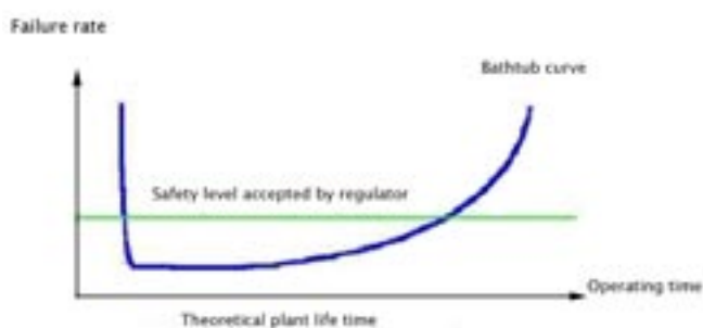
Figure 1: Courbe typique du taux d'incidents en fonction du temps (Meyer, 1998)
