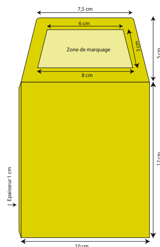
Emplacement pour 2 Ethylotests Etui livré vide
