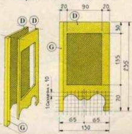
croquis 3-les côtés du buffet
