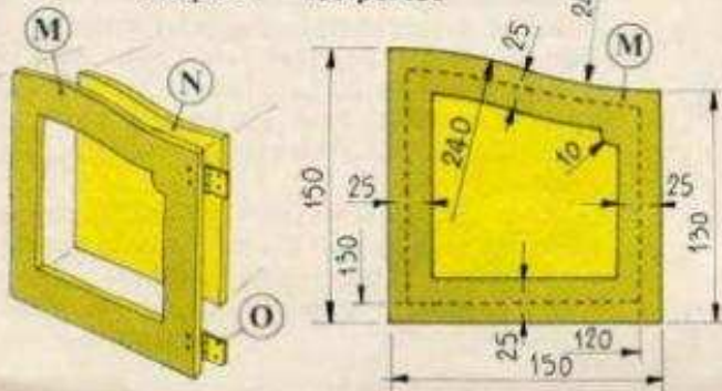
croquis 4 - les portes
