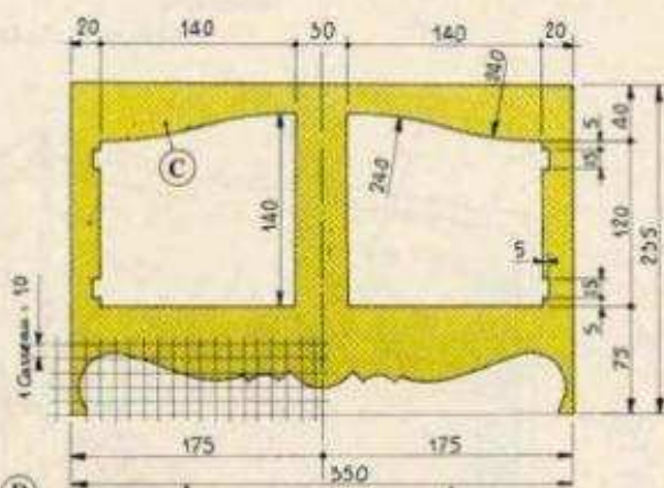
croquis 2-la façade
