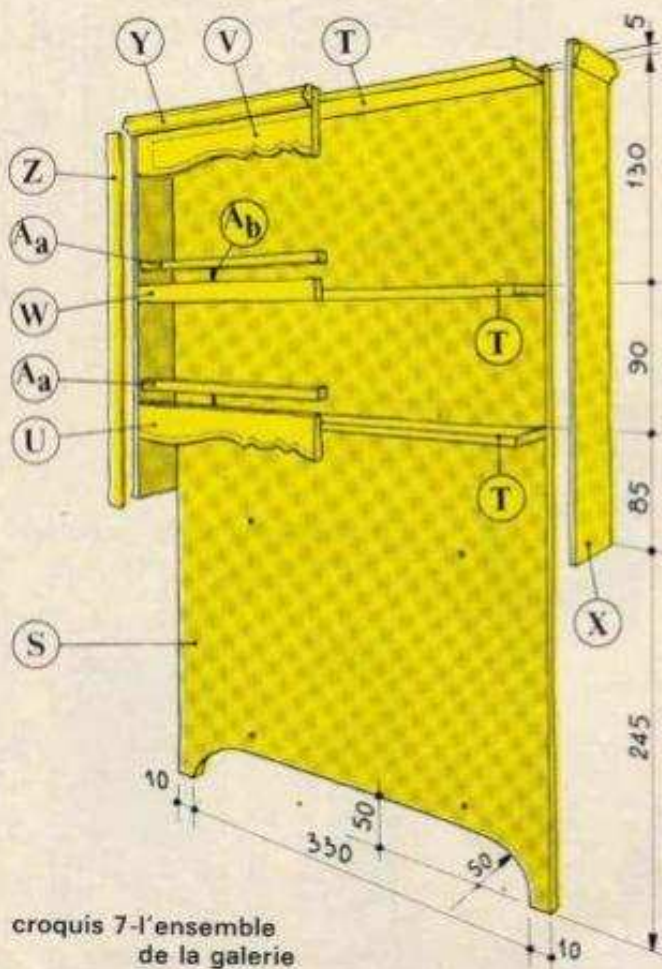
croquis 6 - l'intérieur du buffet
