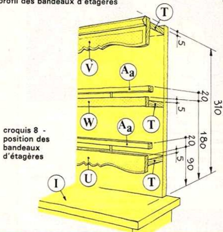
croquis 9 - profil des bandeaux d'étagères
