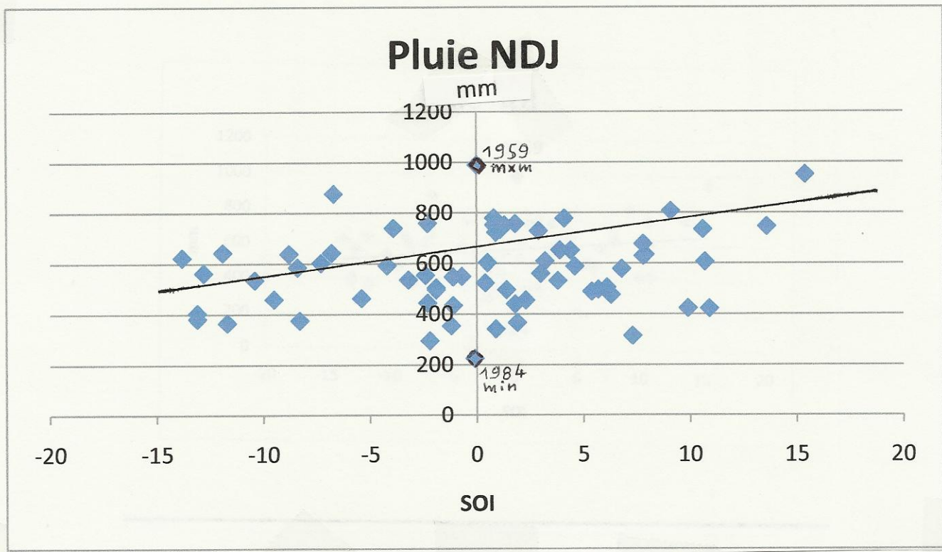
SOI et pluie annuelle à N'Djamena
